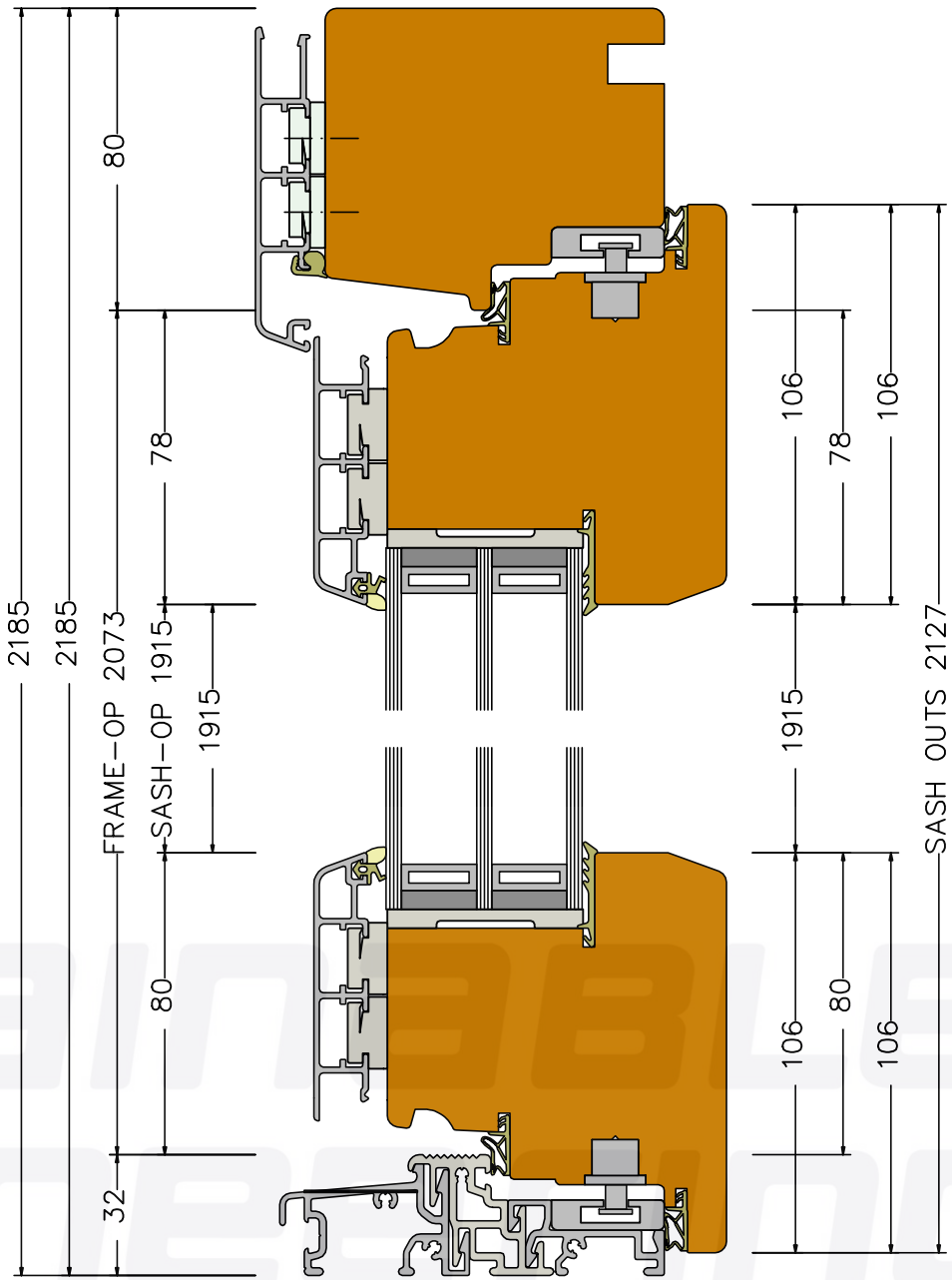
Section V1 (scale 1:2)
