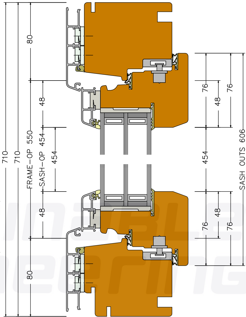
Section V1 (scale 1:2)
