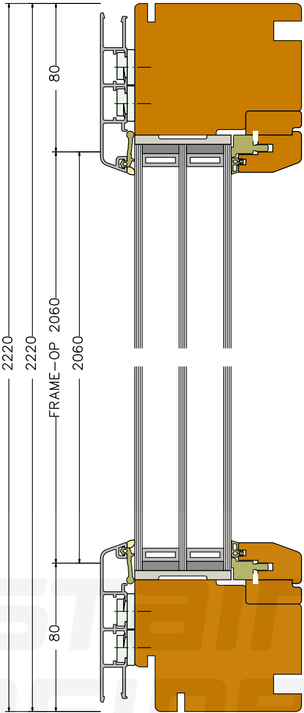
Section V1 (scale 1:2)
