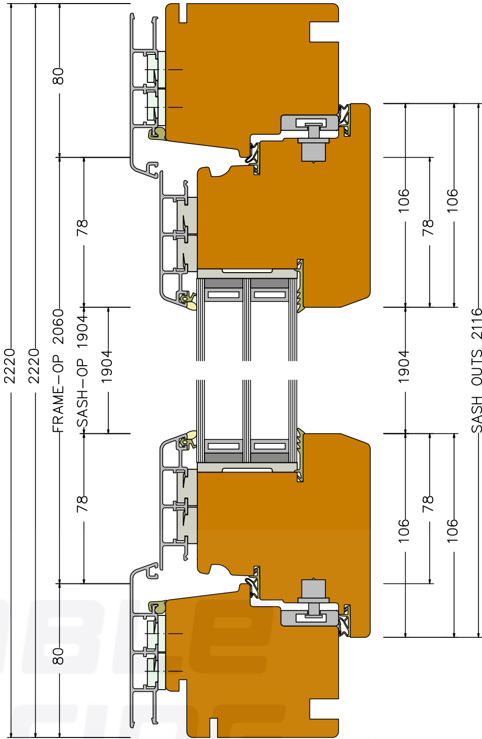
Section V2 (scale 1:2)
